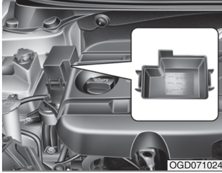
Motor bölümü sigorta paneli (Dizel motor)
